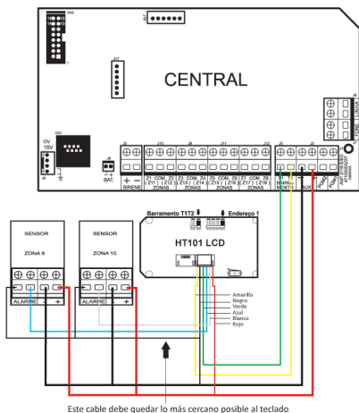
Esquema de conexión del teclado HT101 LCD
